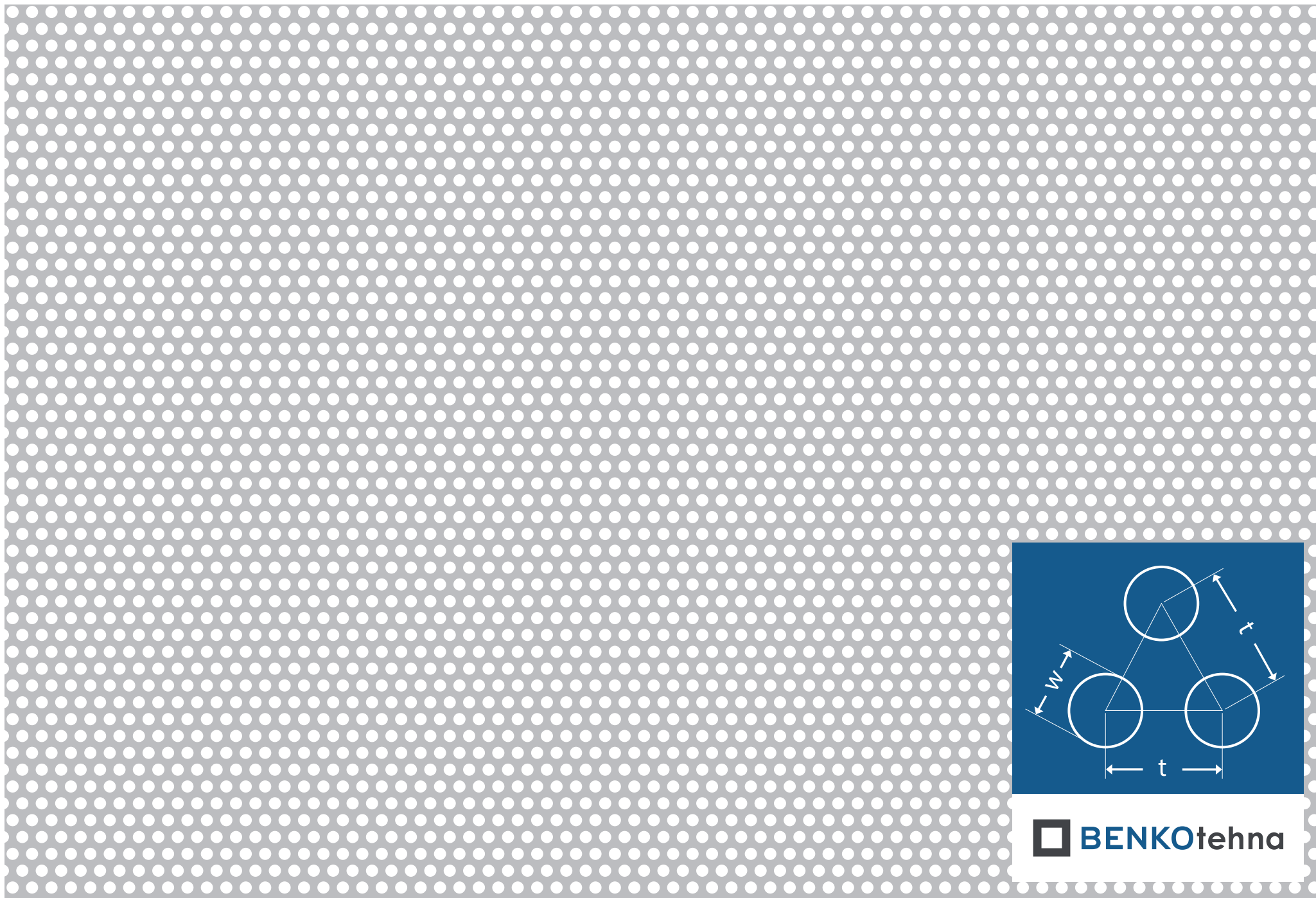
Okrogla zamaknjena Oz 2,5-4: w = 2,5 \text{ mm} | t = 4,0 \text{ mm} | odprtost = 35,43%
