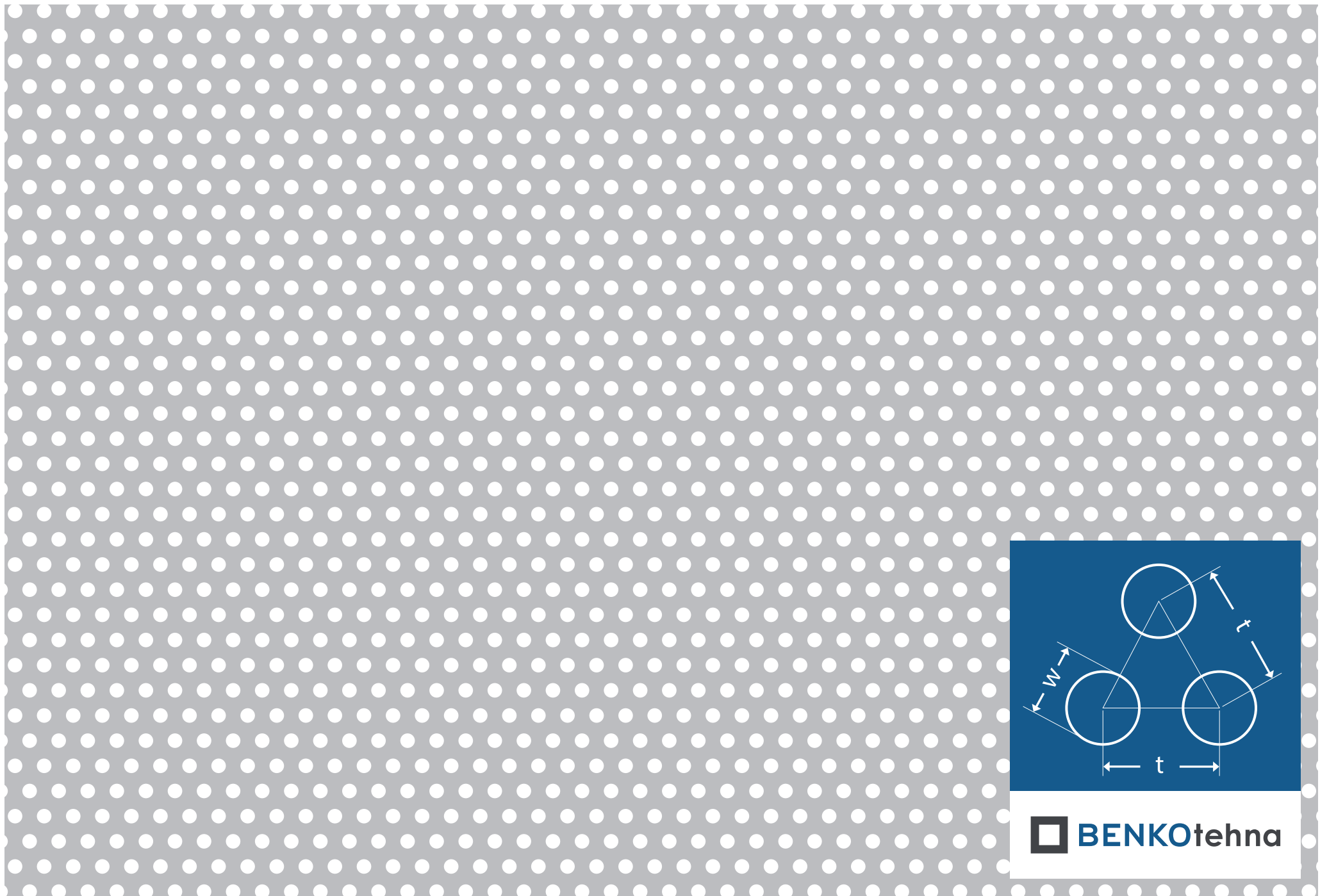
Okrogla zamaknjena Oz 3-6: w = 3,0 \text{ mm} | t = 6,0 \text{ mm} | odprtost = 22,68%
